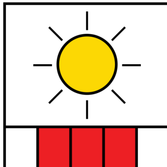
ROTACIÓN
