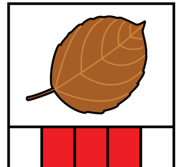
TRASLACIÓN
